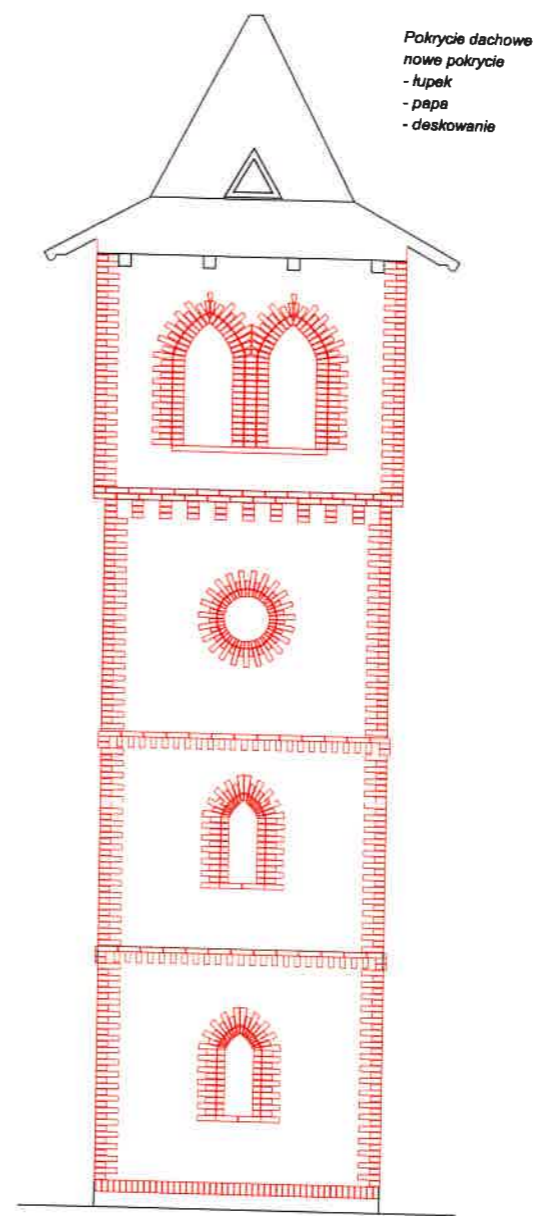
ELEWACJA WIEŻY PÓŁNOCNO-ZACHODNIA
