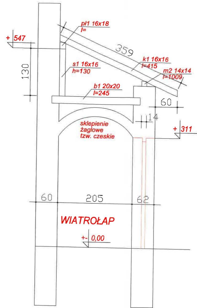
PRZEKRÓJ C-C , D-D
