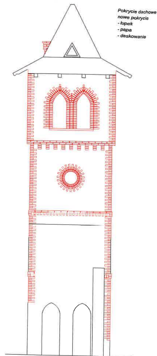
ELEWACJA WIEŻY od strony wejścia POŁUDNIOWO-WSCHODNIA ELEWACJE WIEŻY WIDOKOWEJ
