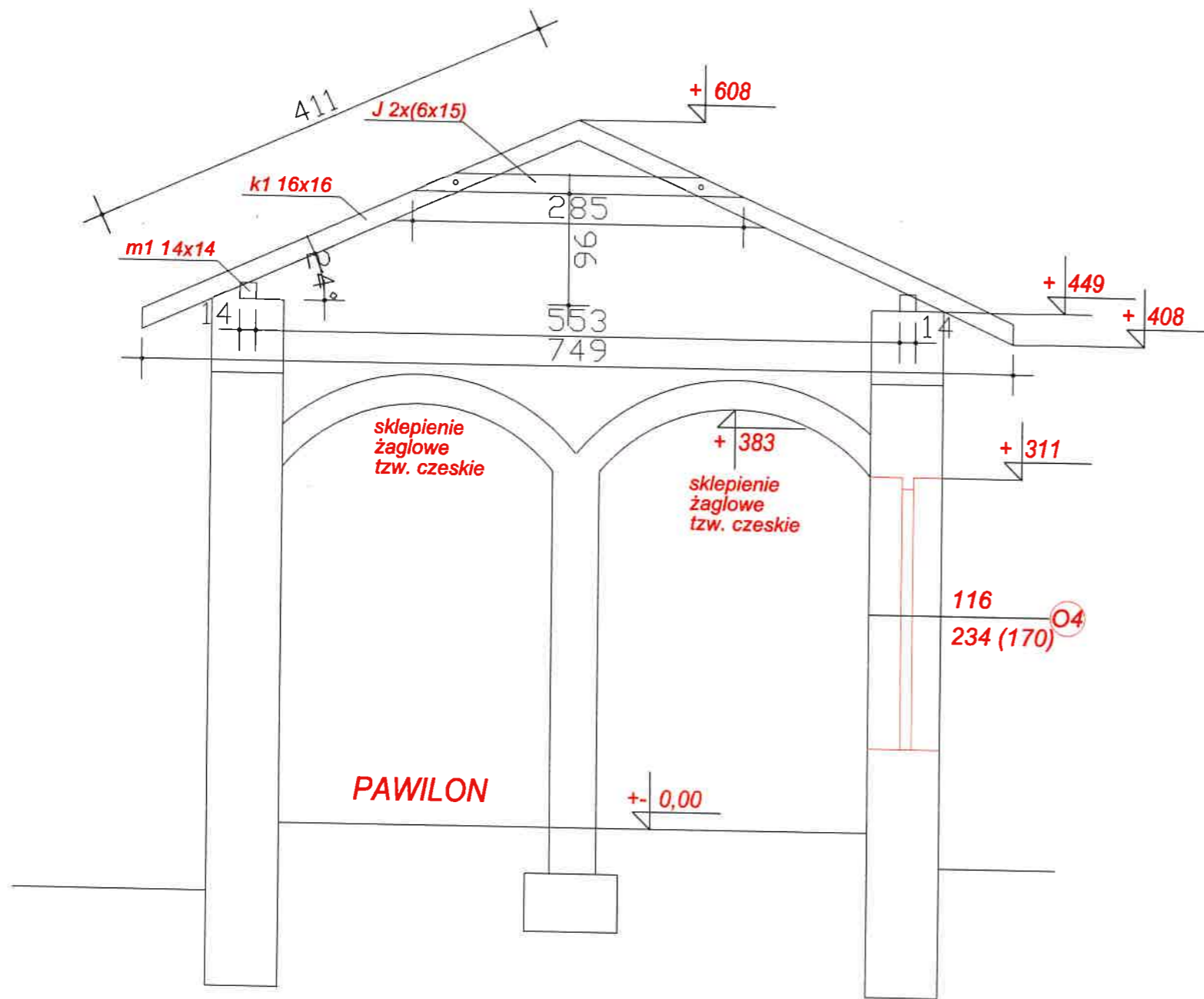
PRZEKRÓJ C-C
